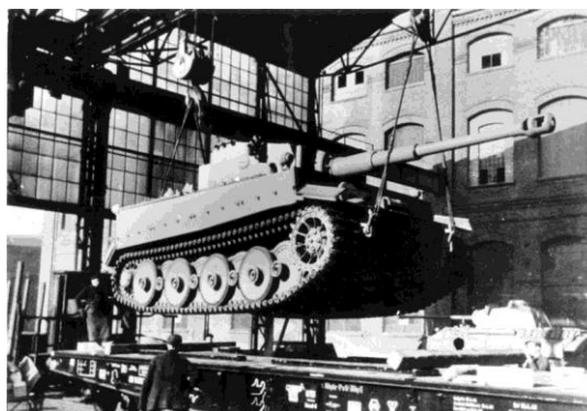
Henschel & Sohn: lo spostamento di un Tiger completo; sullo sfondo si nota un Panzer V Panther
